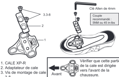
1. XP-R Schuhplatte 2. Schuhplattenadapter 3. 3-8 Schuhplattenschraube Bitte achten Sie darauf, dass die Ausrichtung stimmt
