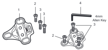
1. XP Placchetta 2. Bullone di Montaggio della Placchetta 3-16D 3. Bullone di Montaggio della Placchetta 3-20 A 4. 4mm Allen Key
