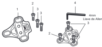
1 XP-R CLEAT 2.3-16D Tornillo de Cleat Mounting 3. 3-20A Tornillo de Cleat Mounting 4. 4mm Llave de Allen
