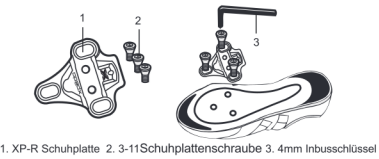
1. XP-R Schuhplatte 2. 3-11 Schuhplattenschraube 3. 4mm Inbusschlüssel
